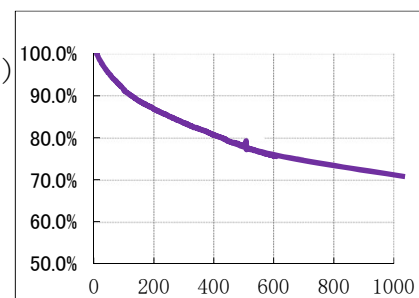
■サイクル特性
